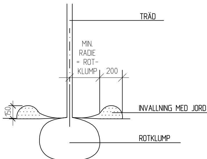
SEKTION SKALA 1:25
